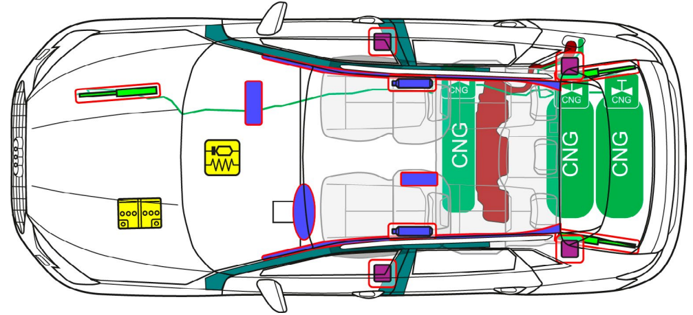
Fiche de secours Audi A3 g-tron (selon ISO 17840)
