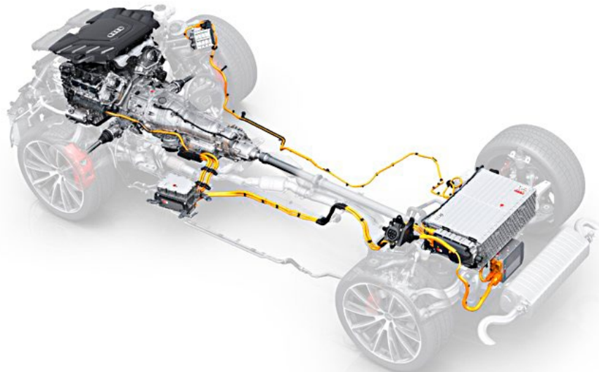
Batterie haute tension à l'arrière du véhicule (Audi Q8 TFSI e)
