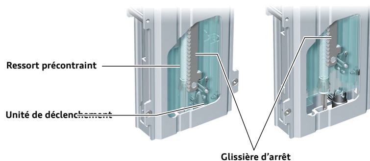
Glissière d'arrêt
