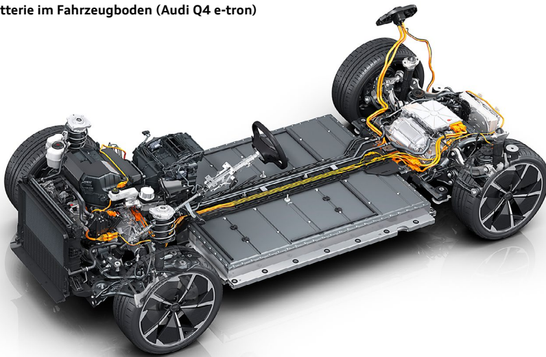
Hochvolt-Batterie im Fahrzeugboden (Audi Q4 e-tron)
