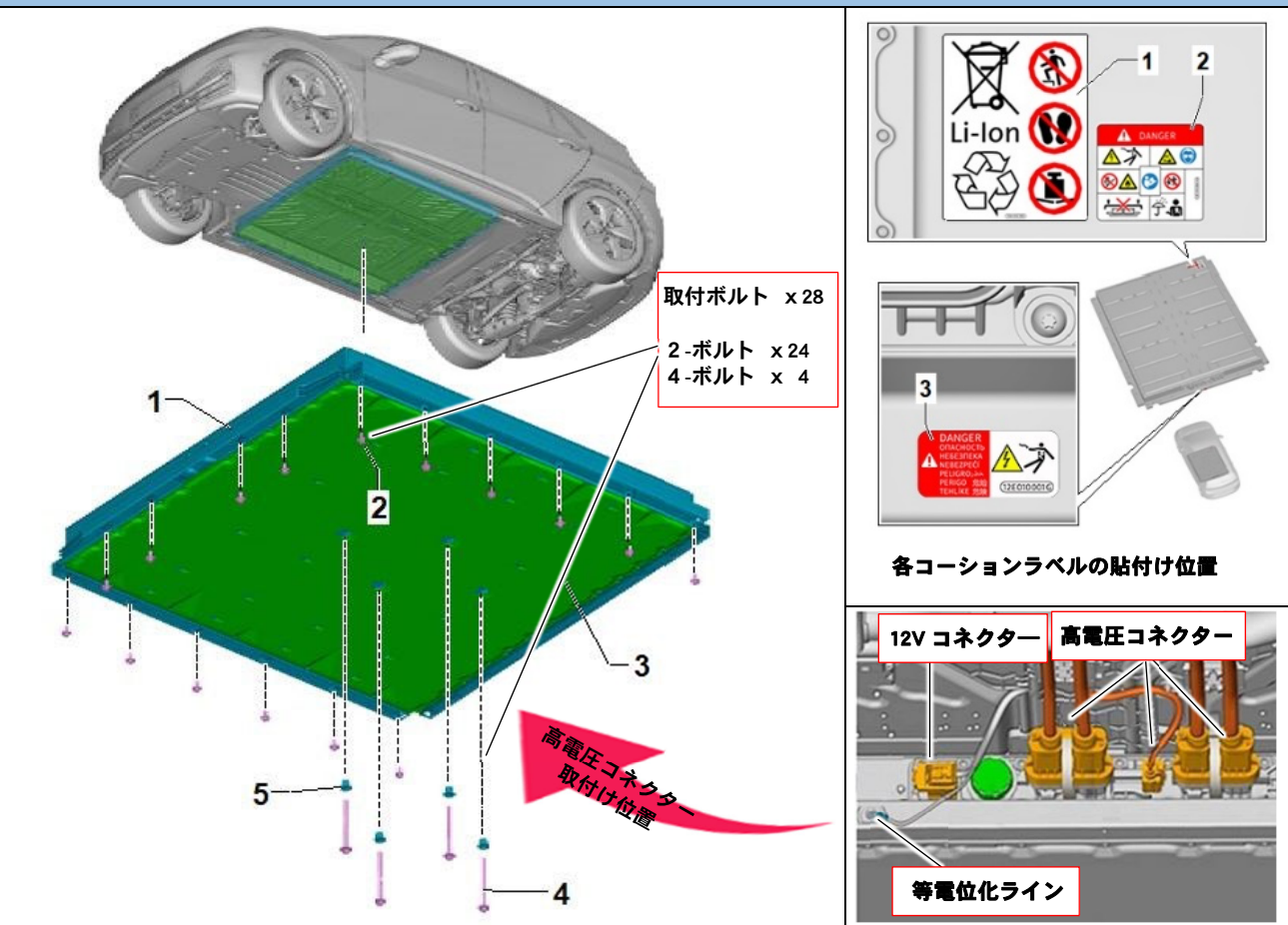
リチウムイオン電池（赤枠は作業か所）
