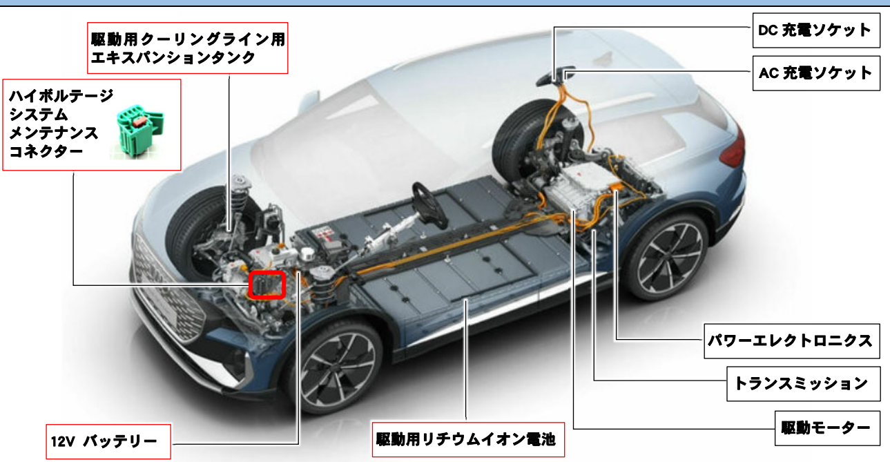
各ユニット配置図（赤枠は作業か所）
